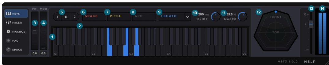
Keys Tab
