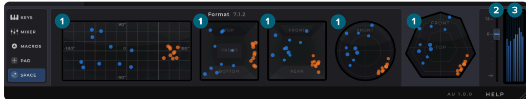
Spatial Tab
